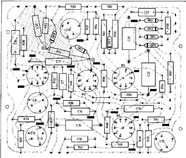
Fig. 2B. Gedrukte-bedradingsplaat A, versterker (onderdelen)
