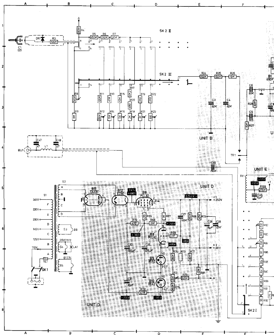
Fig. 36. Circuit diagram GM 6025 - Bild 36. Schaltbild GM 6
