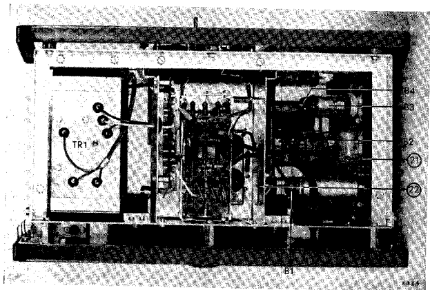
Fig. 26. Onderaanzicht
