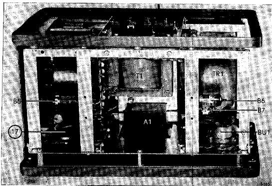
Fig. 24. Bovenaanzicht
