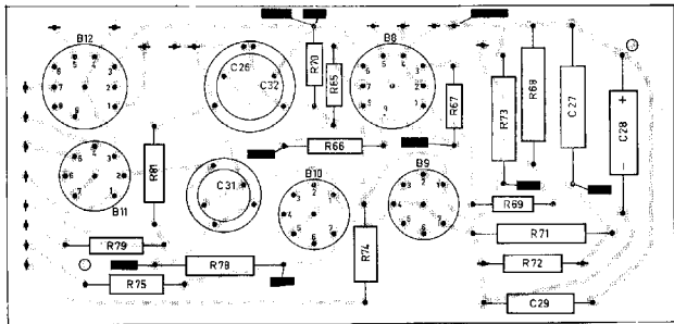
Fig. 31. Gedrukte-bedradsingsplaat D, voedingsdeel
