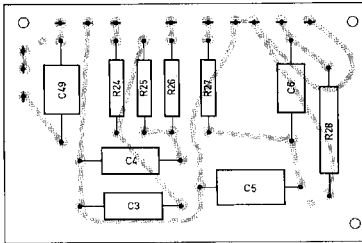
Fig. 30. Gedrukte-bedradsingsplaat B, filter
