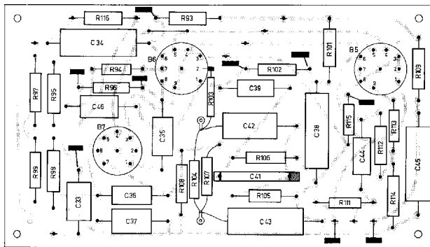
Fig. 32. Gedrukte-bedringsplaat E, ijkspanningsdeel
